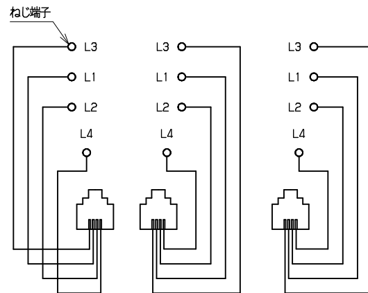
内部接続
