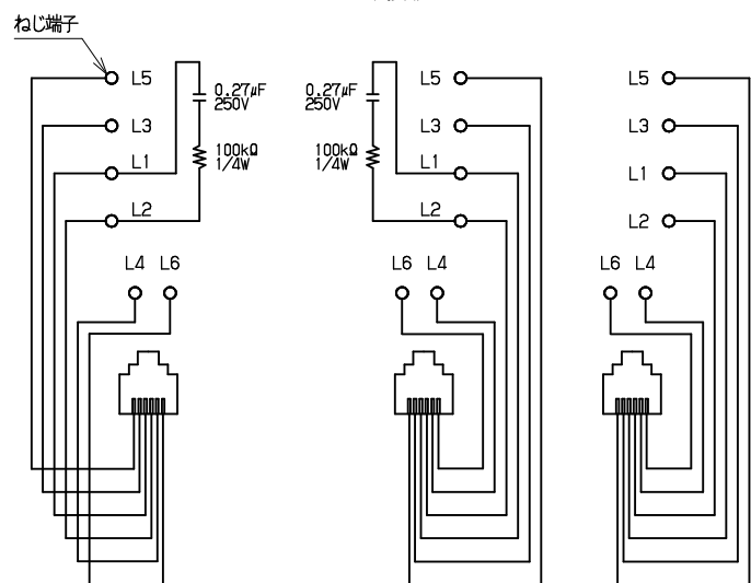
内部接続
