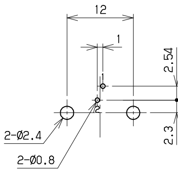
基板取付寸法図 (ジャック取付面)
