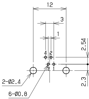
基板取付寸法図 (ジャック取付面)
