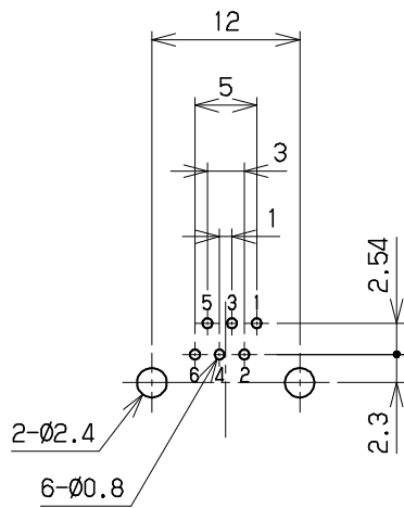
基板取付寸法図 (ジャック取付面)
