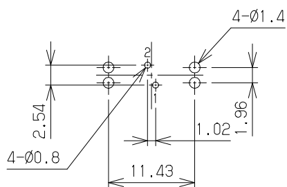
基板取付寸法図 (ジャック取付面)
