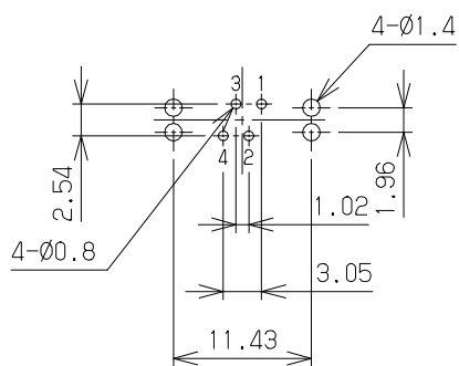
基板取付寸法図 (ジャック取付面)
