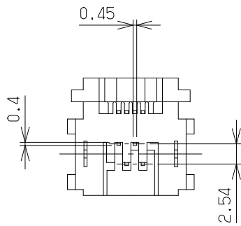
基板取付寸法図 (ジャック取付面)
