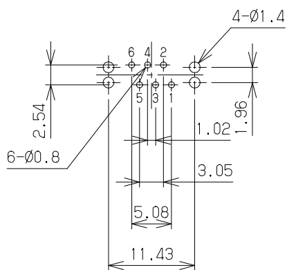
基板取付寸法図 (ジャック取付面)
