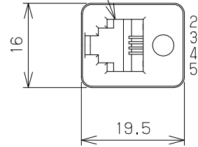
MJ2 (6極 4心)
